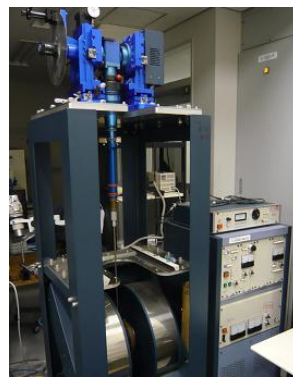
振動試料型磁力計 機器型番：BHV-50
