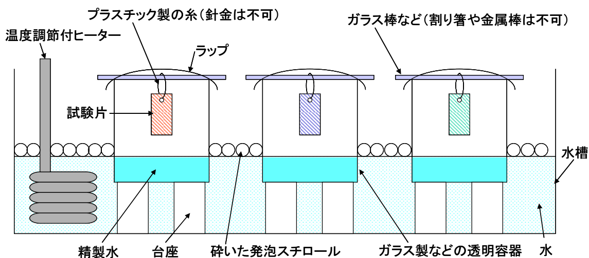
図3 現場で実施できる簡易な加湿試験装置の概略図
